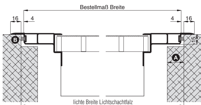
Vertikalschnitt Breite (Vorderansicht)
