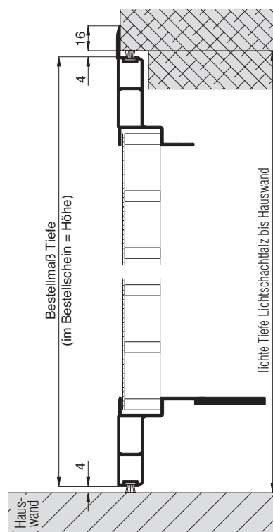
Vertikalschnitt Tiefe (Seitenansicht)
